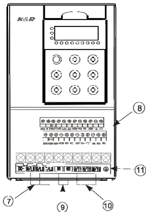
图 2-3 变频器各部位名称示意图
