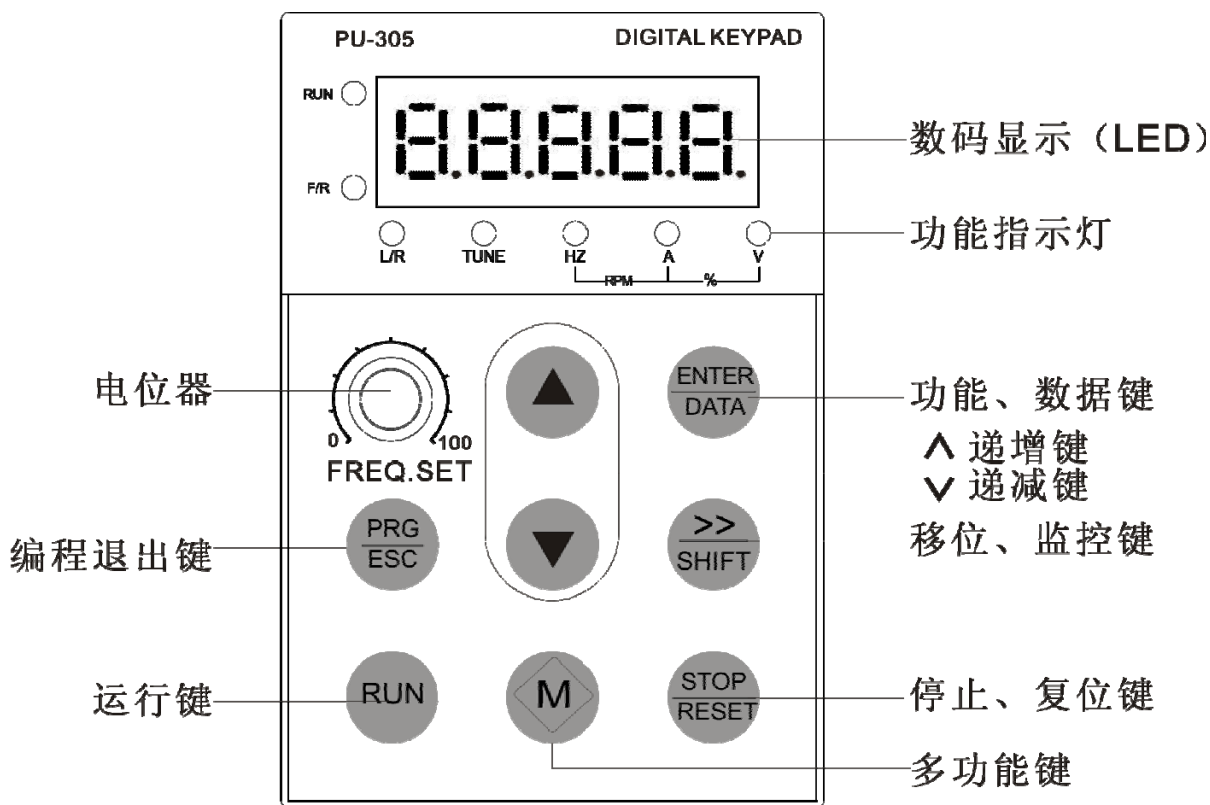
图 4-1 操作键盘示意图
