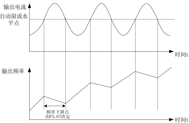
图6-23 限流保护功能示意图
