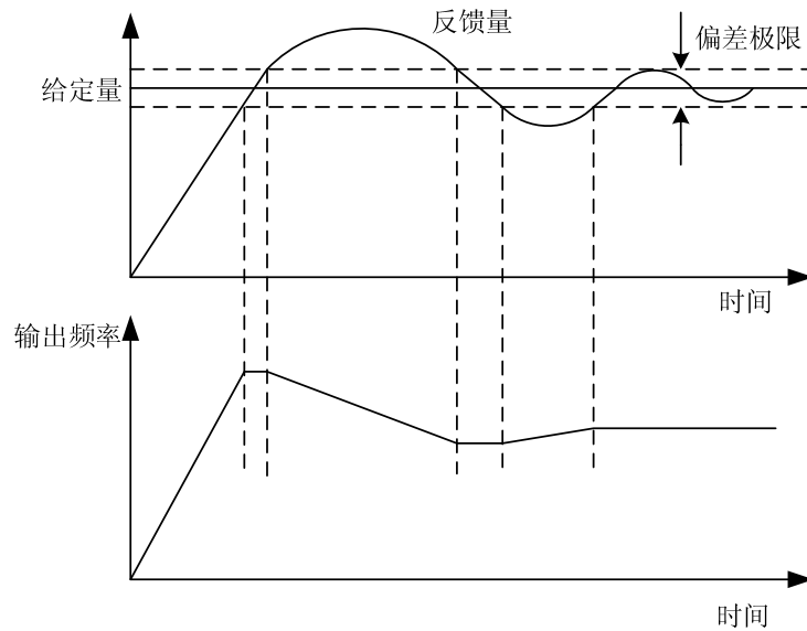
图6-19 偏差极限与输出频率的对应关系
