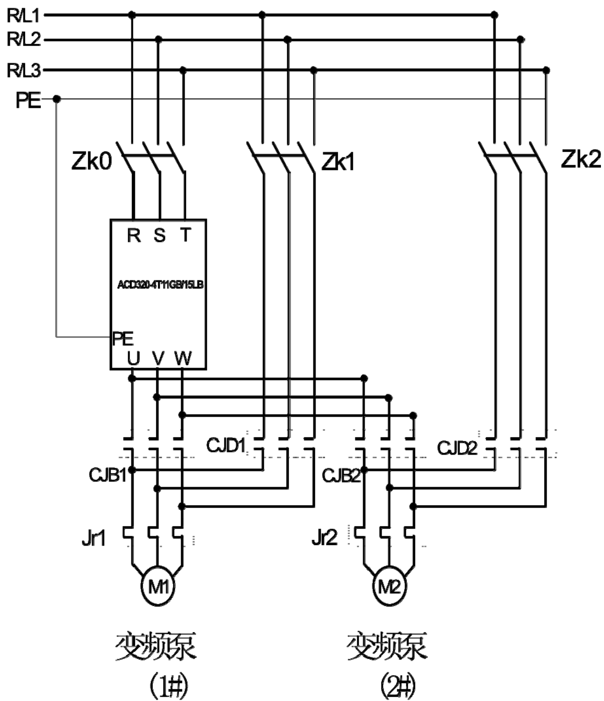
图 9-3 一次连线图
