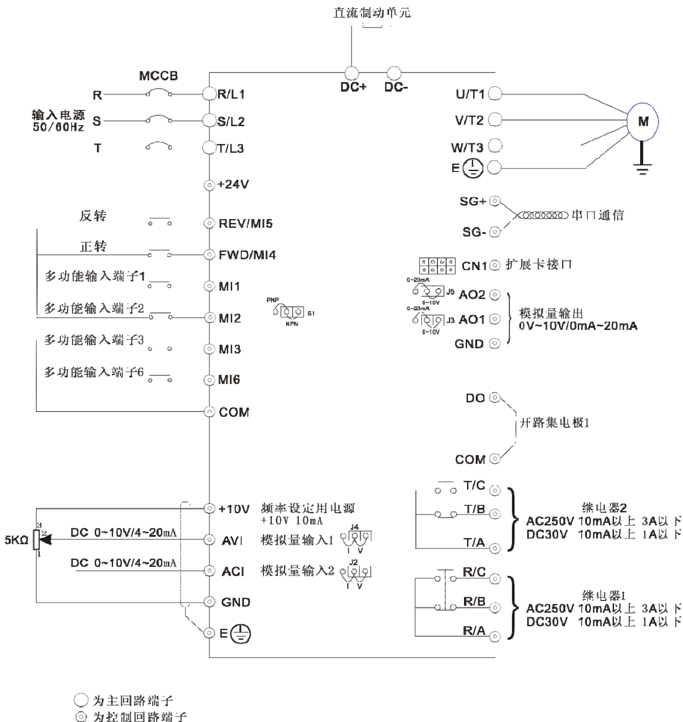
图3-3 主回路端子配线图
