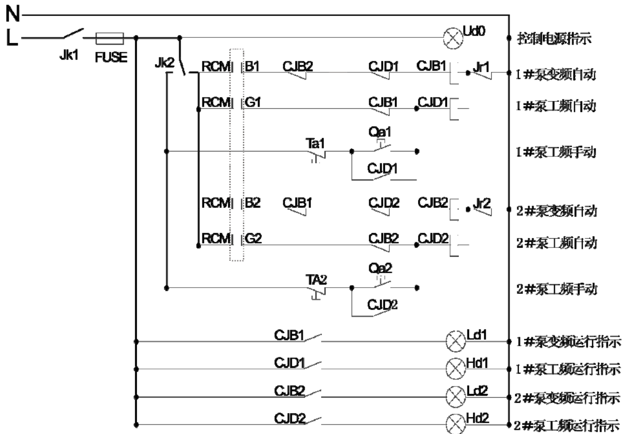
图 9-4 二次连线图
