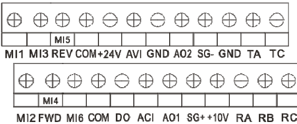
图3-4 7.5KW以下控制端子标识
