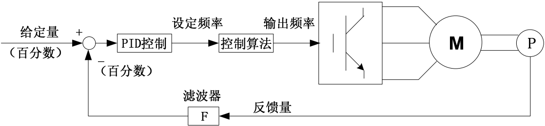
图6 -18 过程PID原理框图
