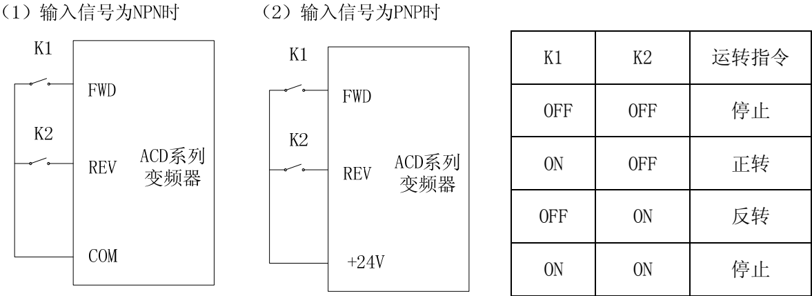
图6-8 两线式运转模式1示意图
