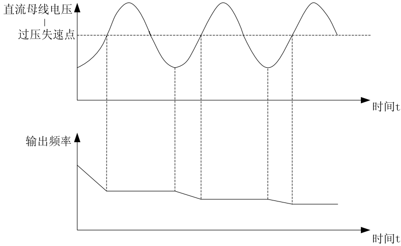
图6-22 过压失速功能
