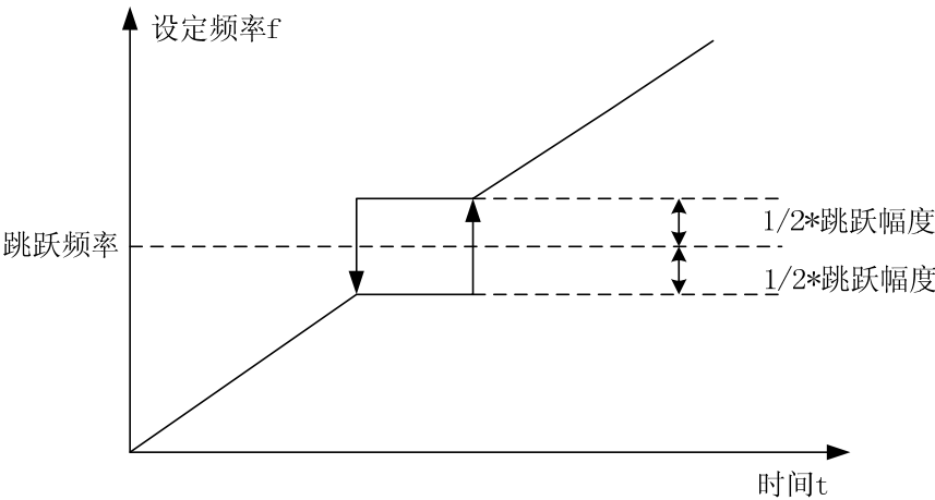
图6-14 跳跃频率示意图
