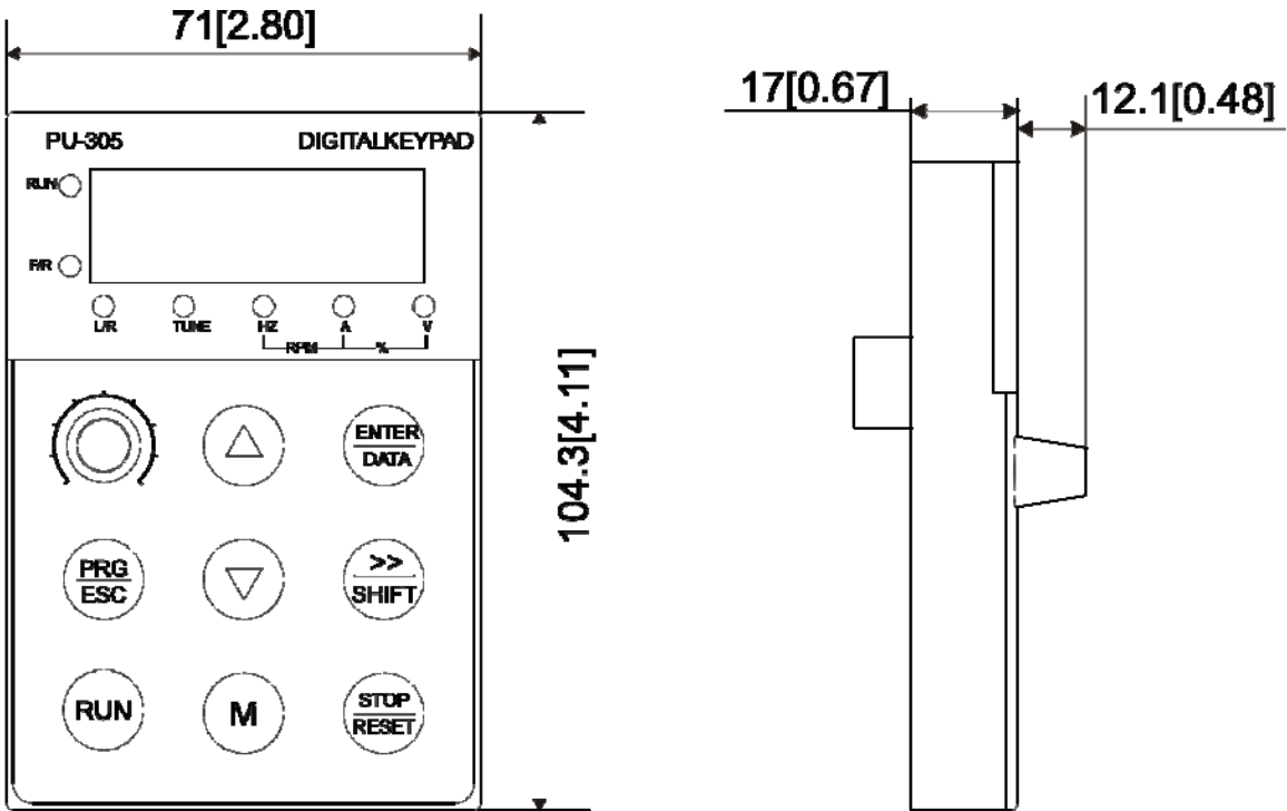
图 2-4 a 外形图
