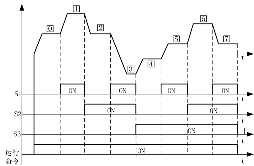
图6 - 20 多段速度运行逻辑图
