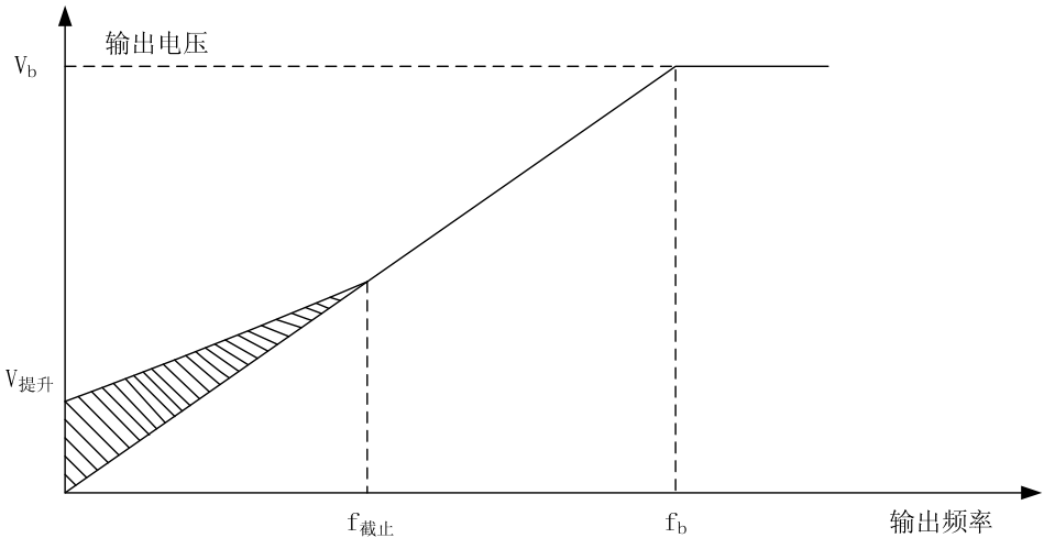
图6-7 手动转矩提升示意图
