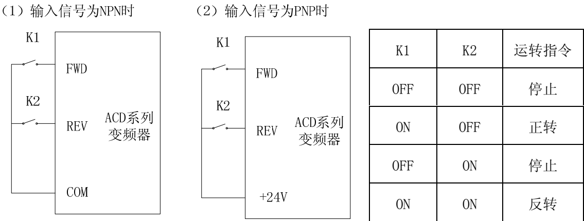
图6-9 两线式运转模式2示意图
