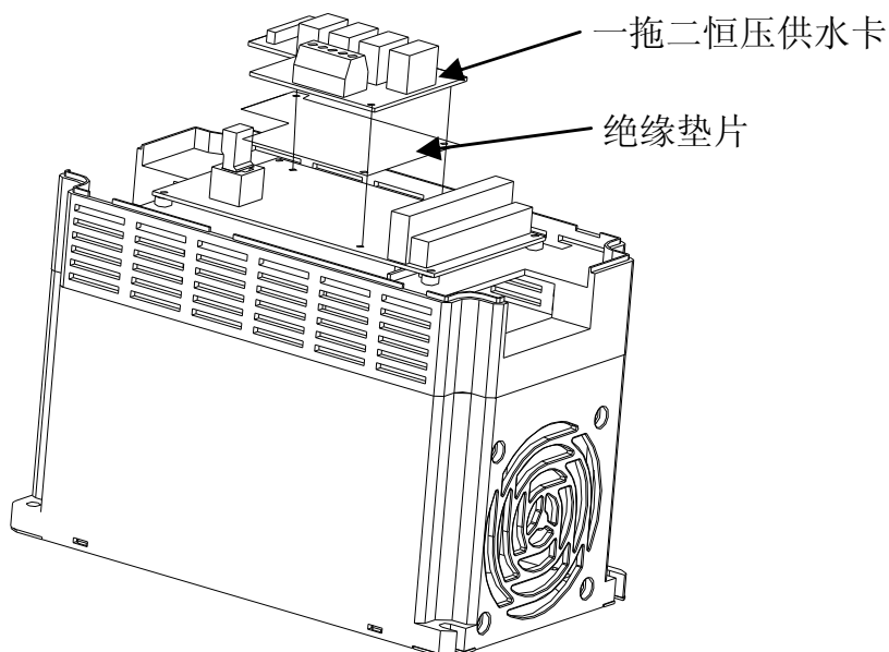
图 9-1 一拖二恒压供水卡安装示意图
