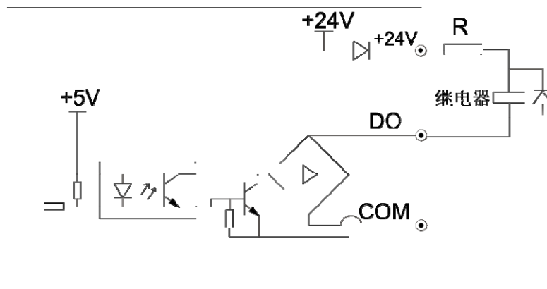
图3-13 数字输出端子接线示意图
