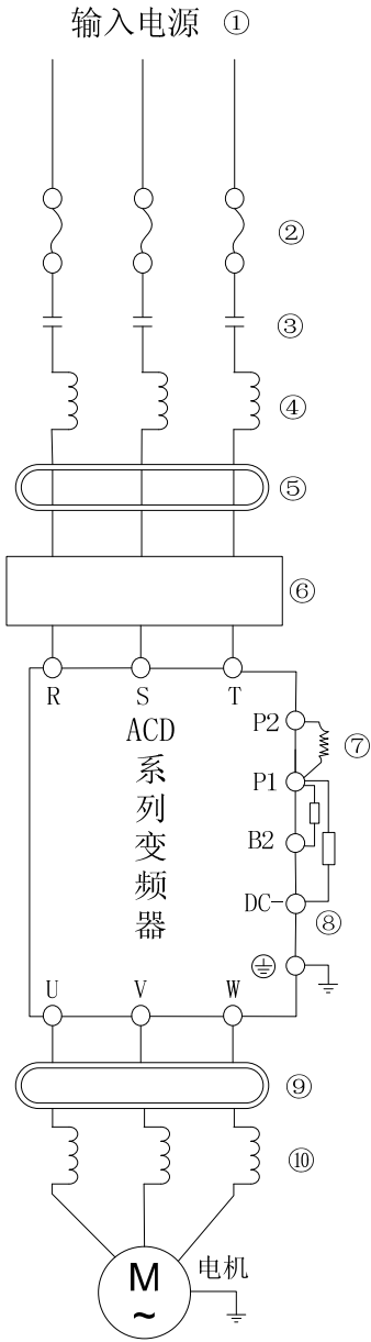
图 3-2 周边设备配线
