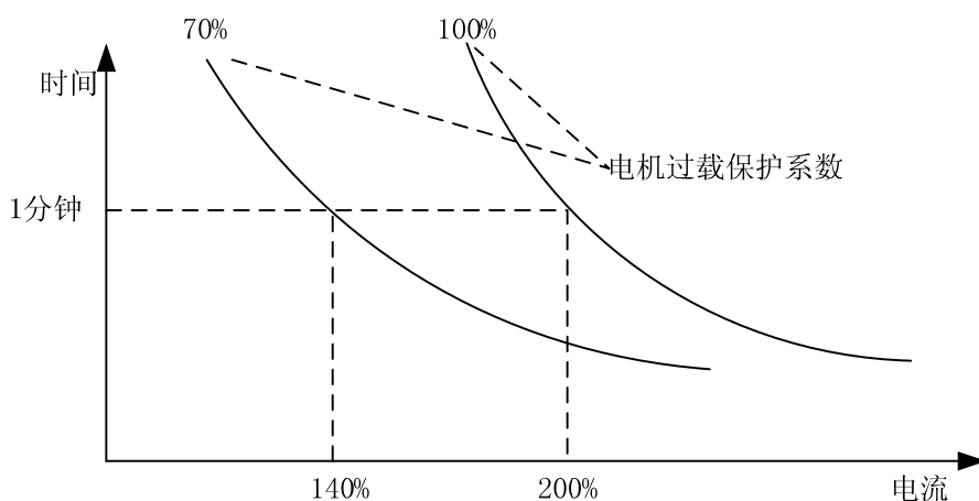
图6-21 电机过载保护系数设定
