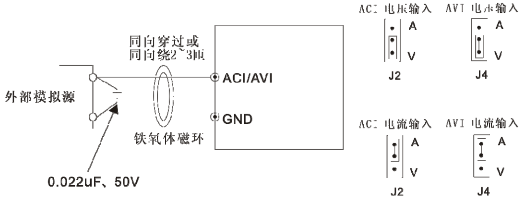
图 3-7 AVI/ACI 端子处理接线图
