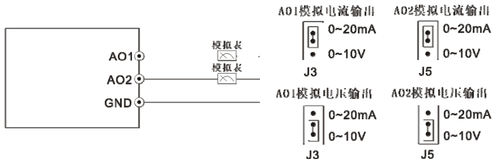
图 3-8 模拟输出端子配线
