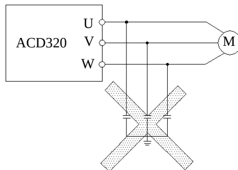
图 1-2 变频器输出端禁止使用电容器
