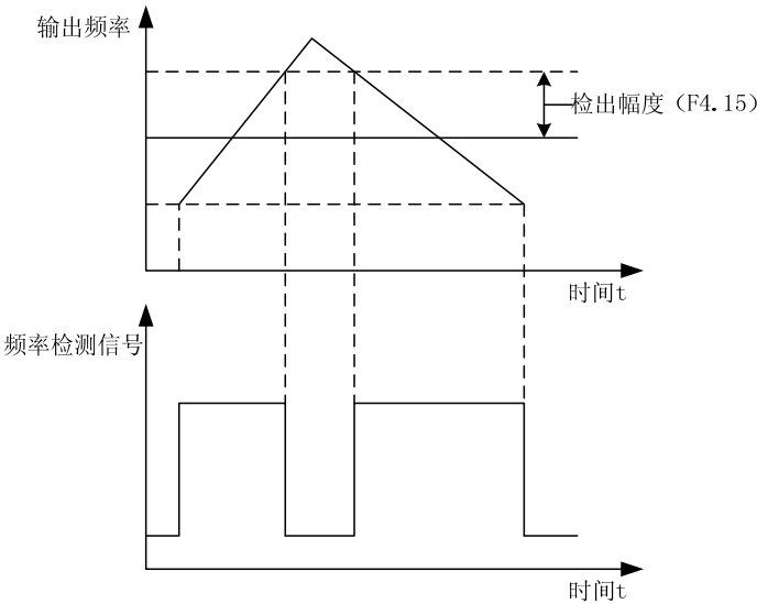
图6-17 频率到达检出幅值示意图
