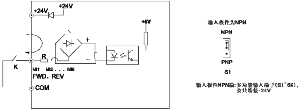
图3—9 使用内部+24V电源的源极的连线方式
