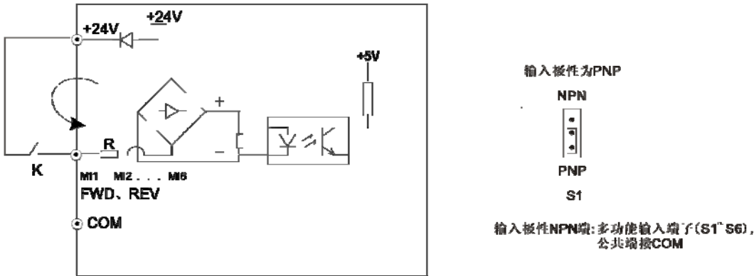
图3—10 使用内部+24V电源的漏极的连线方式
