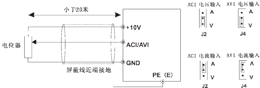
图 3-6 AVI/ACI 端子接线示意图
