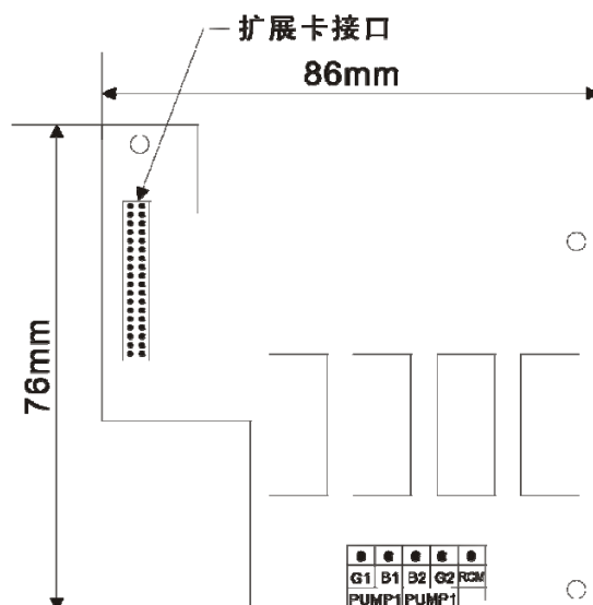
图 9-2 一拖二恒压供水卡外形尺寸示意图
