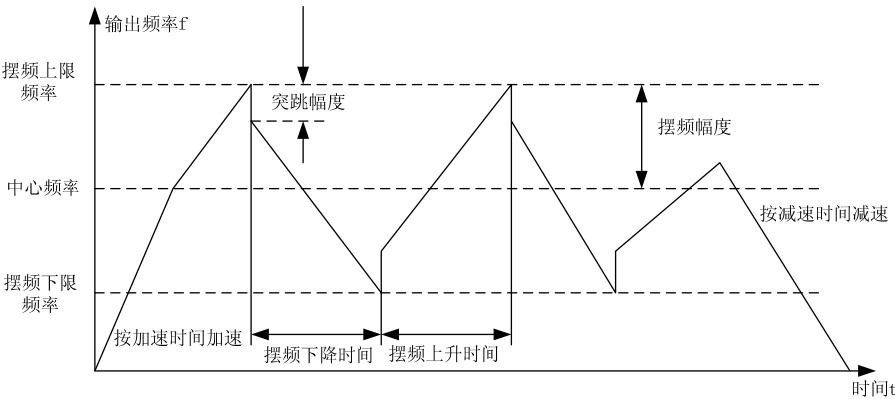
图6-15 摆频运行示意图
