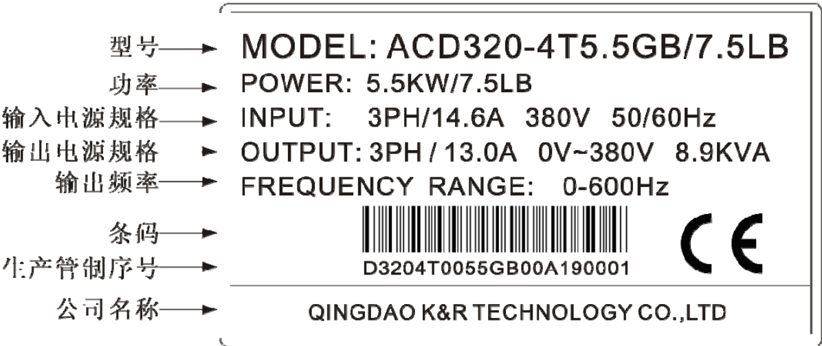
图 2-2 变频器铭牌
