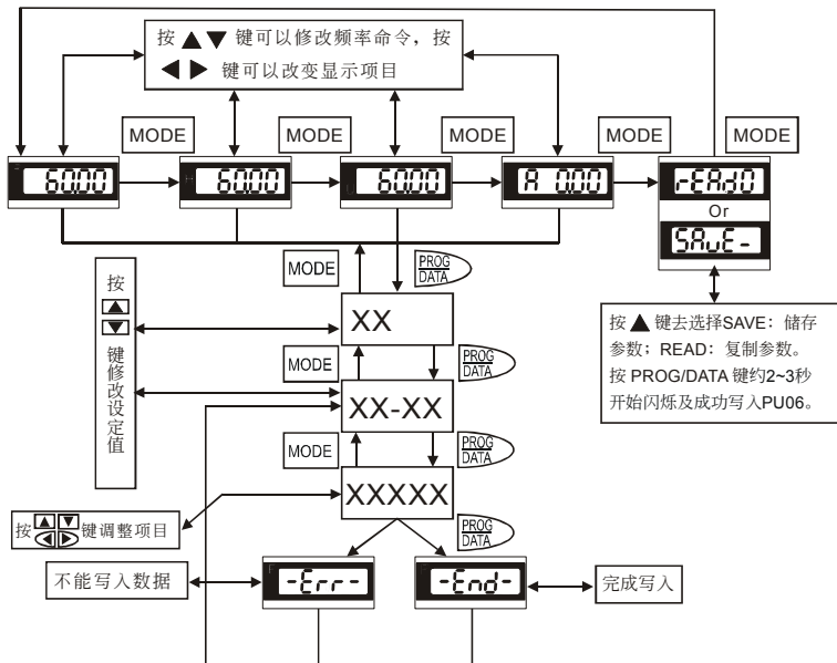
VFD-PU06 操作流程
